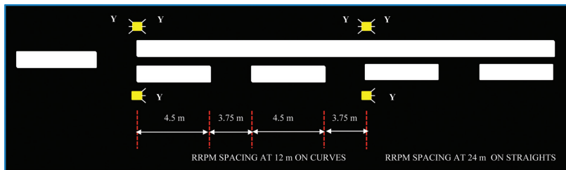
Pemasangan road stud di garis zon larangan memotong.
