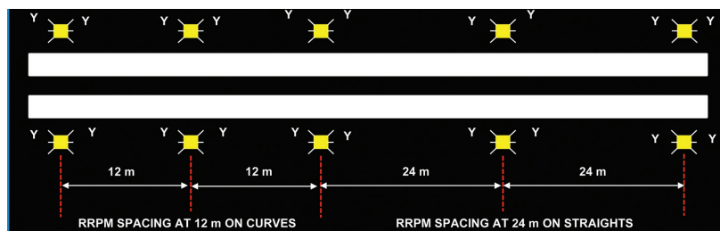
Pemasangan road stud di sepanjang laluan selekoh dan zon larangan memotong.
