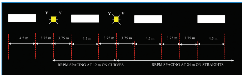
Pemasangan road stud di garis tengah.
