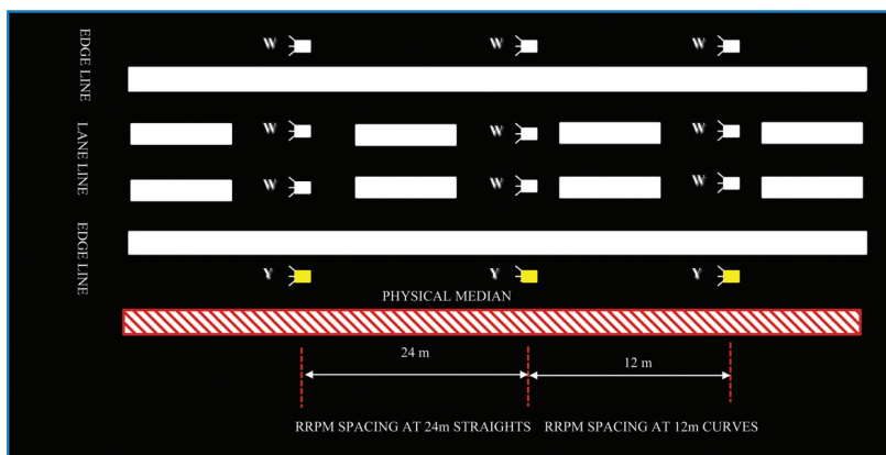
Pemasangan road stud di jalan berkembar.
