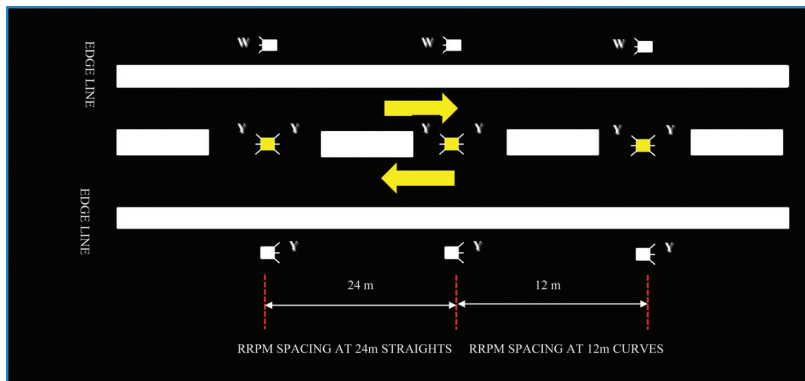
Pemasangan road stud di jalan tunggal.
