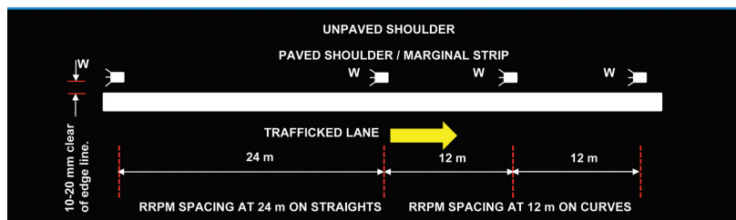
Pemasangan road stud di garisan tepi jalan.
