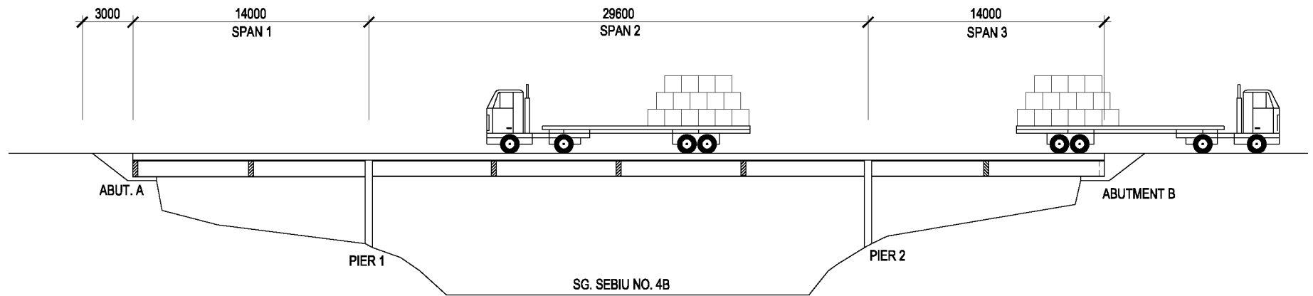
LONGITUDINAL SECTION
