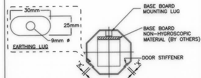
DETAIL 2 : DOUBLE SLOT HINGE SERVICE DOOR
