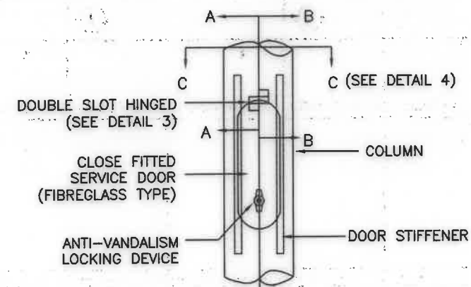
DETAIL 2 : DOUBLE SLOT HINGE SERVICE DOOR
