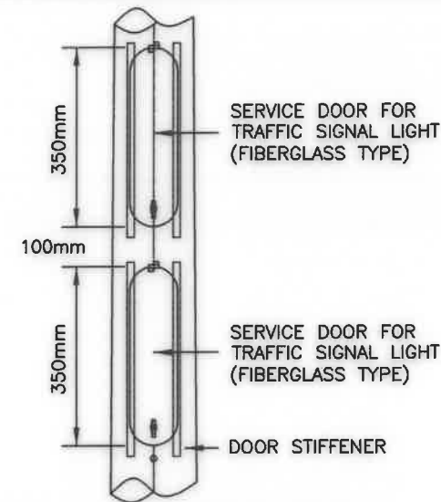
DETAIL 1 : 2 SERVICE DOOR
