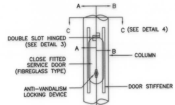
DETAIL 2 : DOUBLE SLOT HINGE SERVICE DOOR
