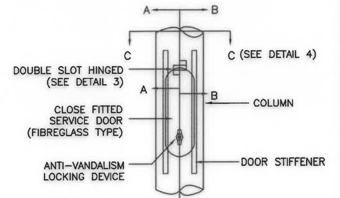
DETAIL 2 : DOUBLE SLOT HINGE SERVICE DOOR
