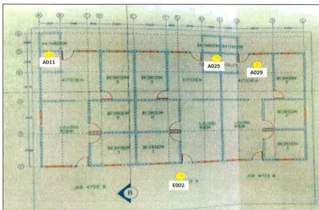
PELAN LANTAI
